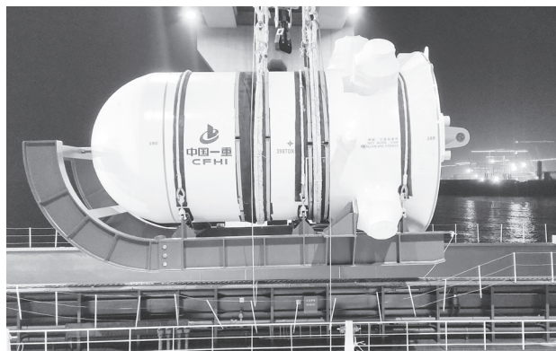
>> “国和一号”反应堆压力容器 国家电投/供图
