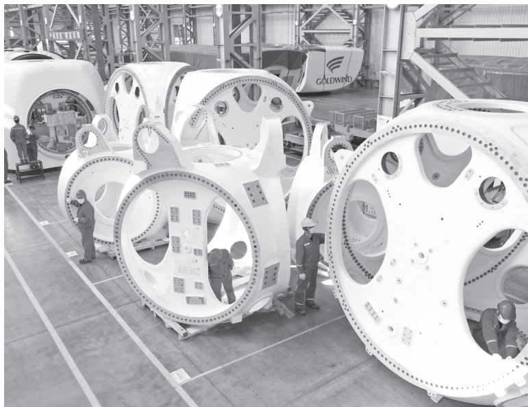
>> 河北省隆化县立足区位优势，打造风电装备制造产业集群，助推经济高质量发展。图为工人在车间装配风电机舱 金良快/摄
