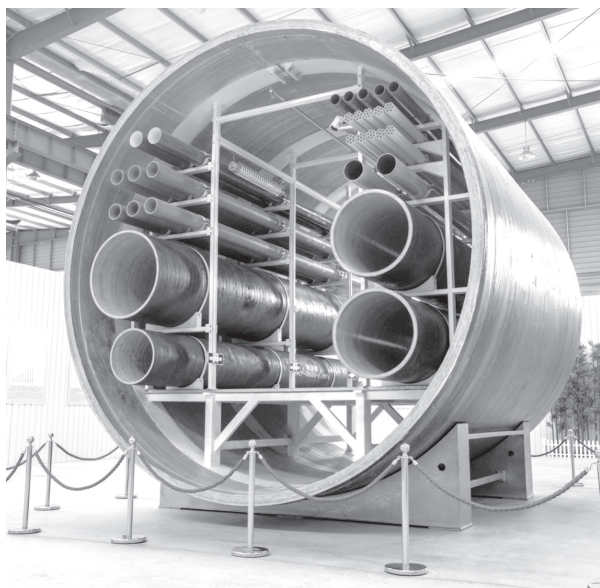
>> 竹缠绕复合管 宋莎莎 / 供图
