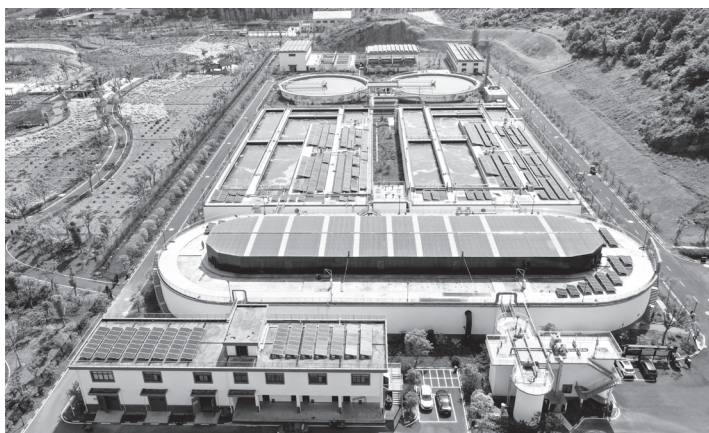
>> 浙江省仙居县城市建设发展集团污水处理厂充分利用厂房屋顶和污水处理池空间，安装太阳能光伏板发电，生产清洁电能，每年可提供约140万千瓦时绿色清洁电能 华文武/摄
