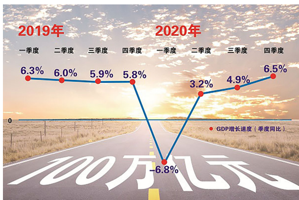
2019至2020年各季度GDP增长速度“V”形曲线 制图：王婵
